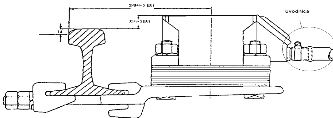
Nosač balize
